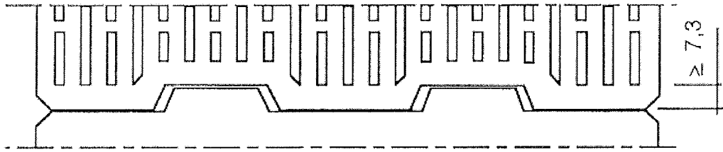
a) Lochbildführung im Bereich Außenquersteg
