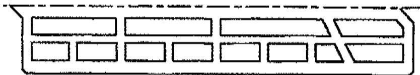
b) Lochbildvariante der äußeren Kernreihe des Delta-Ziegels
