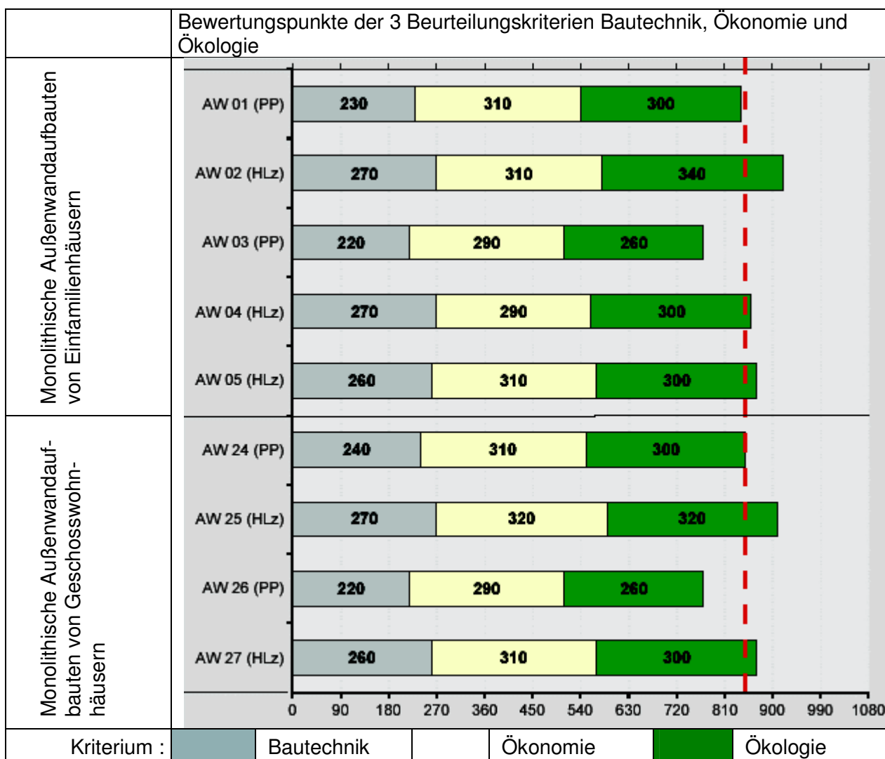
Bild 1: Übersicht der untersuchten monolithischen Außenwandaufbauten, getrennt nach Einfamilien- und Geschosswohnhäusern. Die senkrechte rote Linie stellt die Mittelwerte der erreichten Gesamtpunktzahl von ca. 850 Punkten dar.
