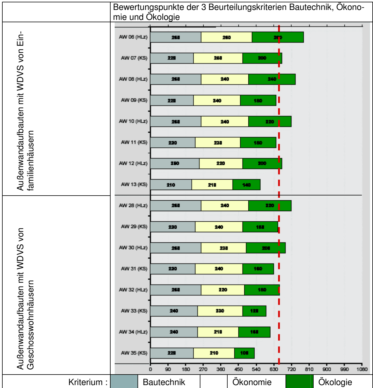
Bild 2: Übersicht der untersuchten Außenwandaufbauten mit WDVS, getrennt nach Einfamilien- und Geschosshäusern. Die senkrechte rote Linie stellt die Mittelwerte der erreichten Gesamtpunktzahl von ca. 650 Punkten dar.
